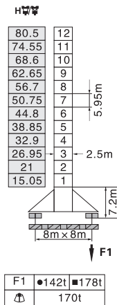
行走式 Traveling
