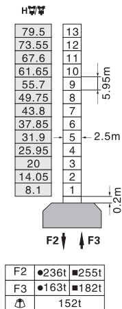
固定式 Stationary
